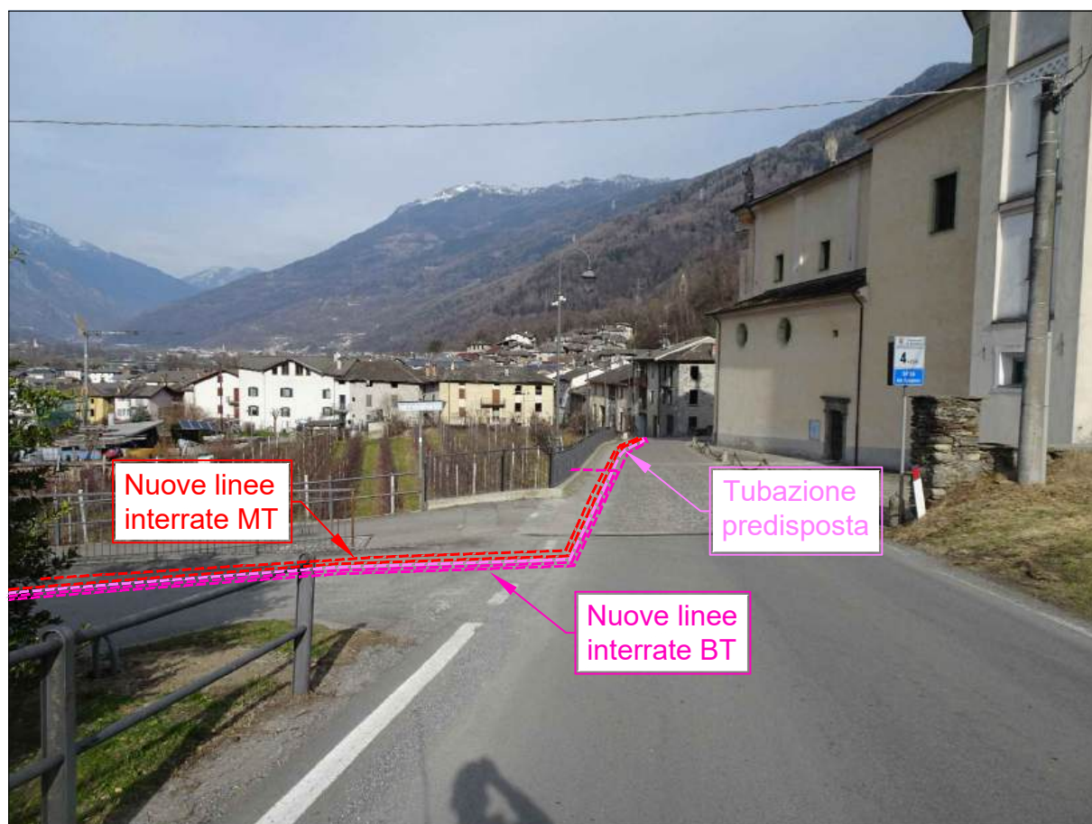
FOTO 8: VIA PROVINCIALE (S.P. n°26) POSA NUOVA LINEA INTERRATA MT
