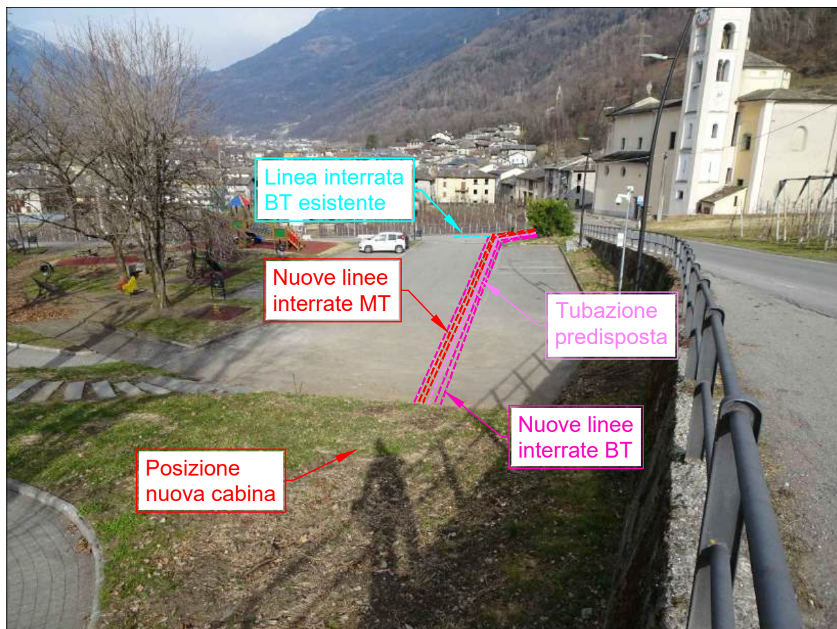
FOTO 7: PARCHEGGIO E VIA PROVINCIALE (S.P. n°26) POSA NUOVA LINEA INTERRATA MT
