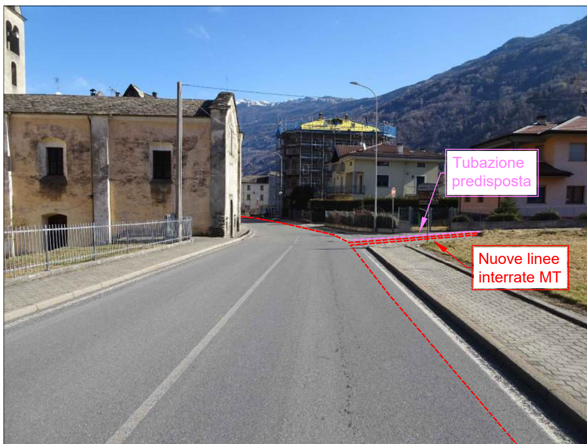
FOTO 2: VIA ROMA (S.P. n°27) POSA NUOVA LINEA INTERRATA MT
