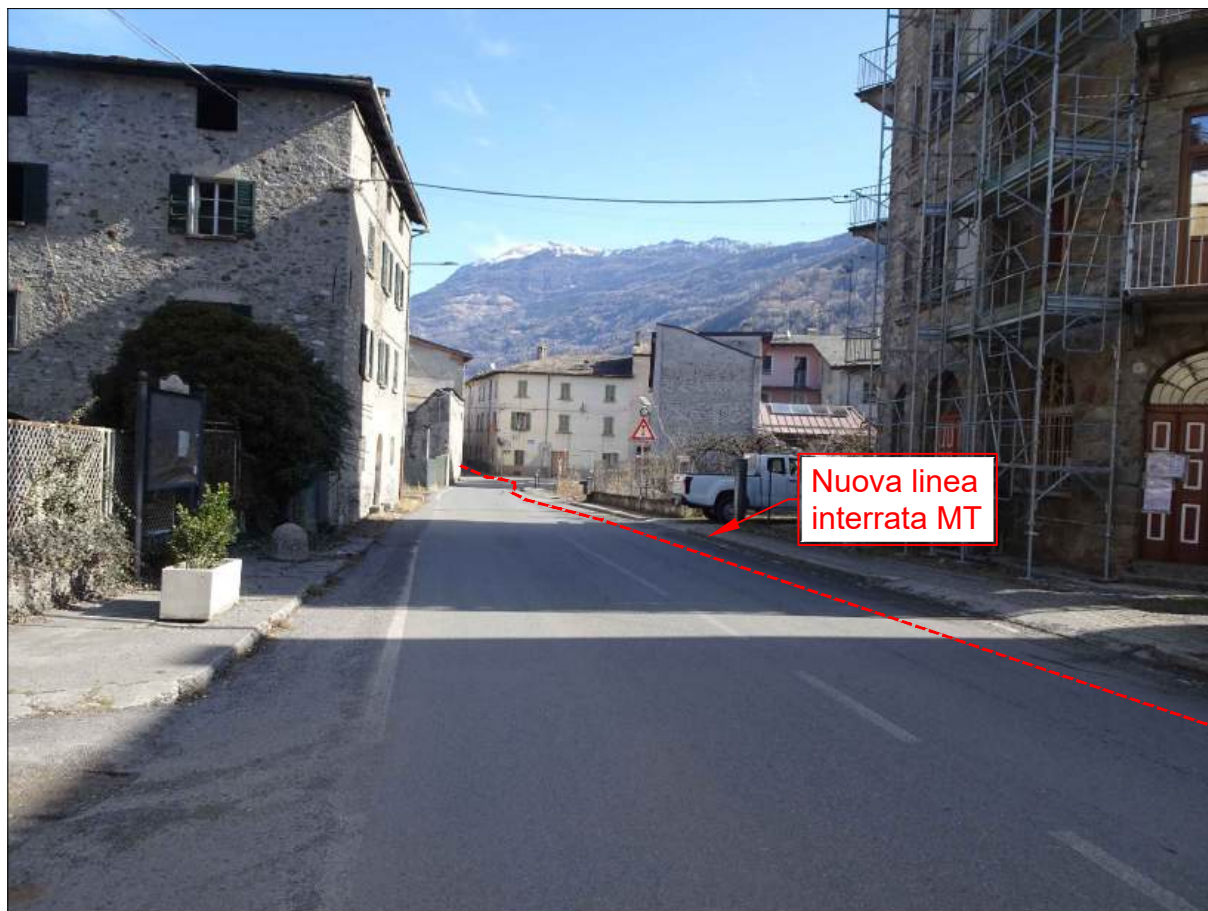
FOTO 3: VIA ROMA (S.P. n°27) POSA NUOVA LINEA INTERRATA MT
