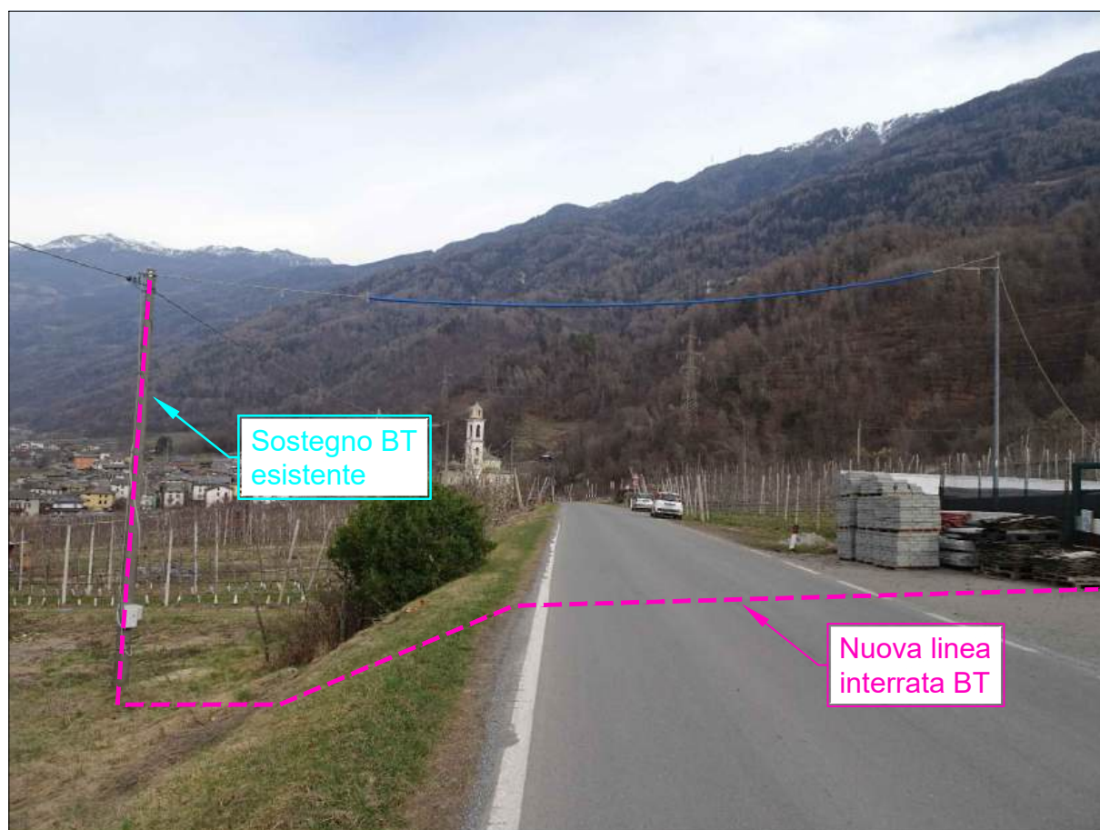
FOTO 6: VIA PROVINCIALE (S.P. n°26) POSA NUOVA LINEA INTERRATA BT
