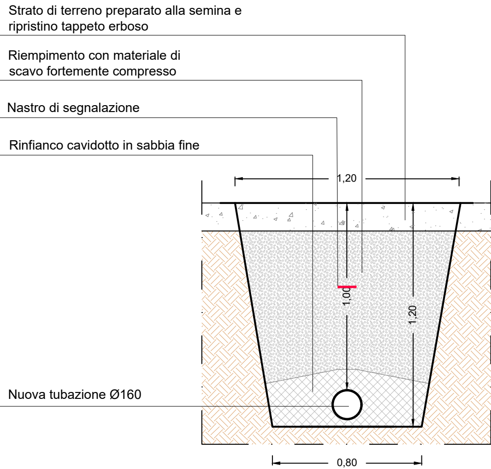
PARTICOLARE SEZIONE DI SCAVO SU STRADA -Scala 1:20- PARTICOLARE SEZIONE DI SCAVO SU VERSANTE -Scala 1:20-
