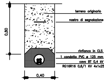
SEZIONE TRATTO (H-I)
