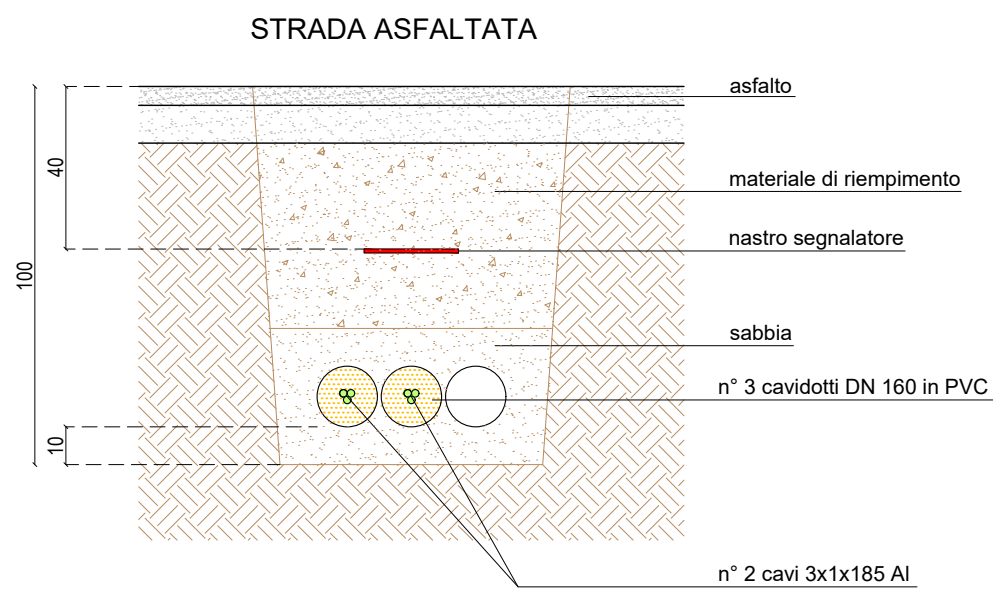
SEZIONI TIPO DI SCAVO - scala 1:20
